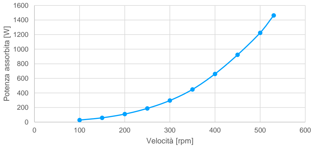
Grafico Velocità vs Potenza assorbita
